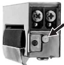
Elektrozaczep tradycyjny serii 1400
