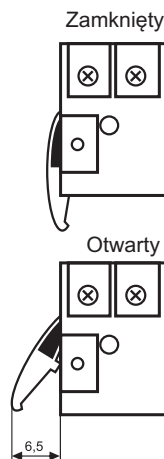
Elektrozaczep tradycyjny serii 1400
